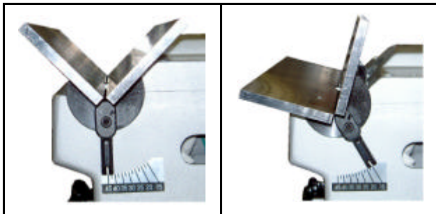
Chamfering Angle 45 °
