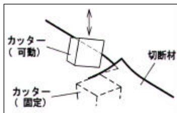
刃部構造図
