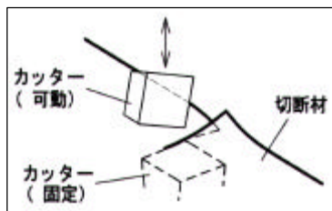
刃部構造図
