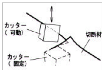
刃部構造図
